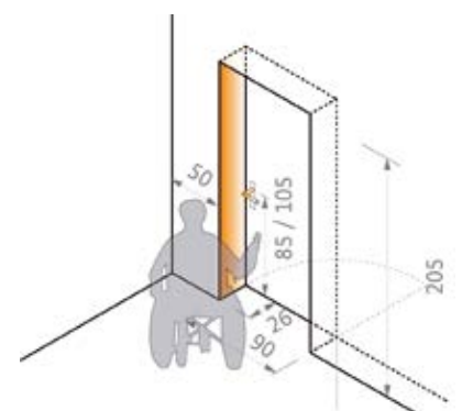
Türmaße
