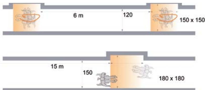
Geometrie der inneren Erschließung nach DIN 18040-1:2010-10
