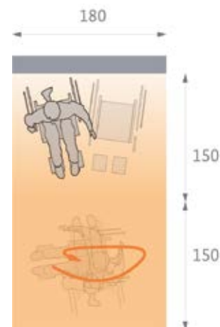
Flächenbedarf Rollstuhlwechsel
